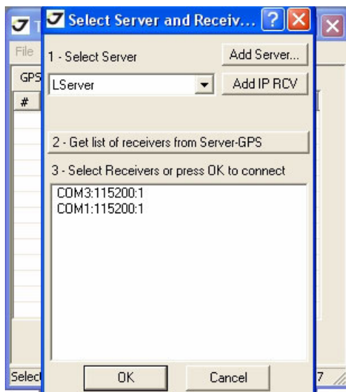
Рисунок 3-6. Параметры соединения
