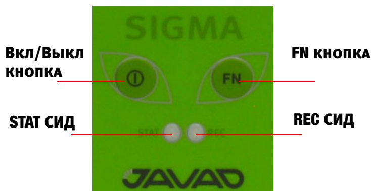
Рисунок 3-14. TriPad
