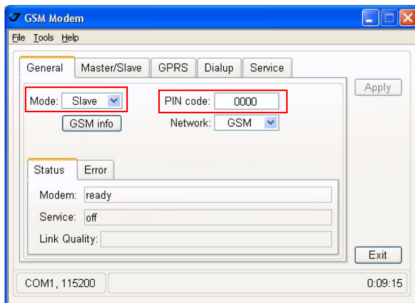
Рисунок 3-4. Закладка General
