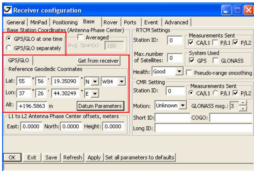
Рисунок 3-10. Закладка Base
