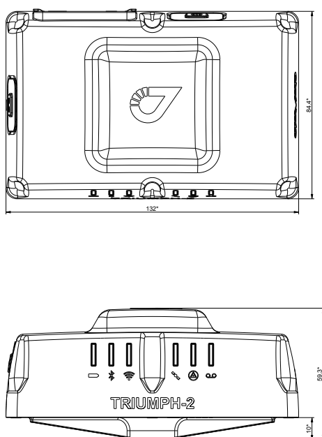
Рисунок 2. Габариты ТРИУМФ-2
