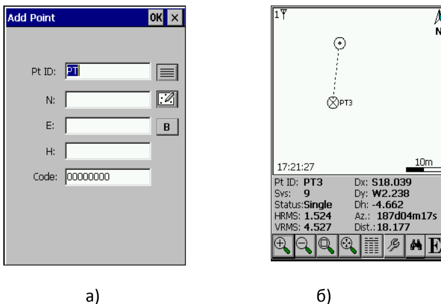
Рис.6.14 Вынос точки в натуру
