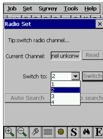
Рисунок 5.13 Окно выбора радиоканала
