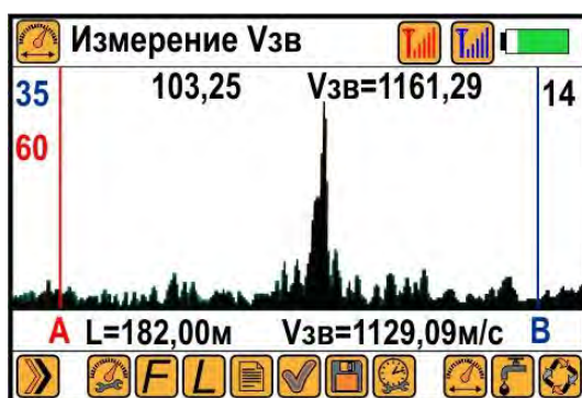
Рисунок 14 Измерение скорости звука
