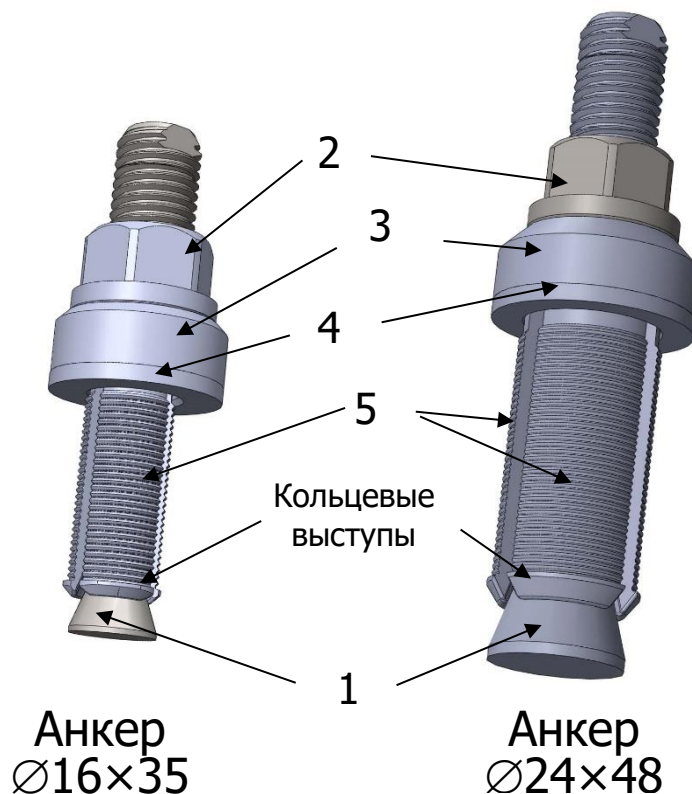
Рисунок 2 – Анкерные устройства (анкера) в сборе
